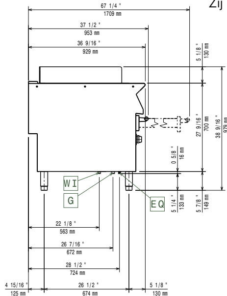
Zij aanzicht
